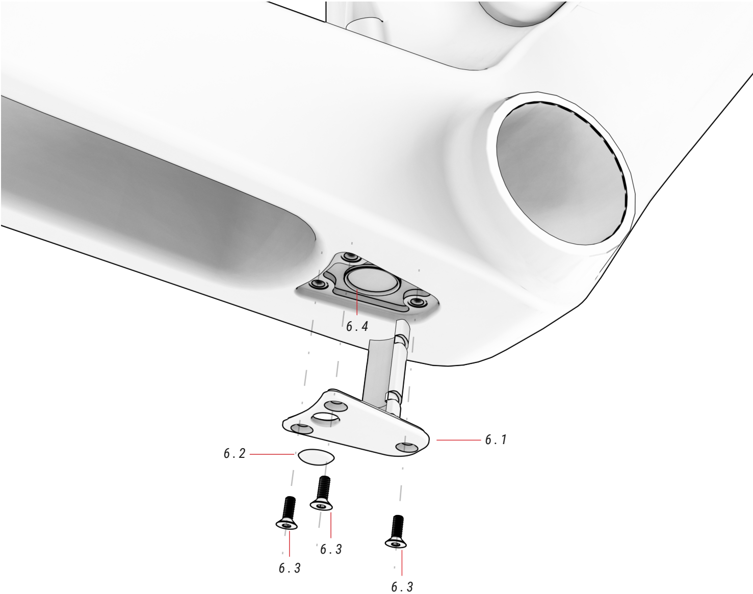
06 KOMORA AKUMULATORA ref.: 381548100
