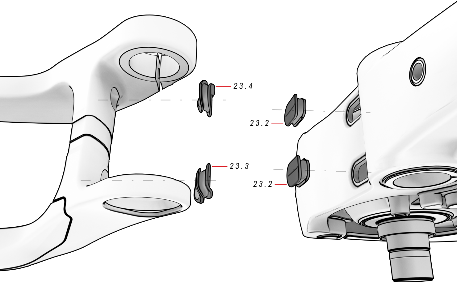
23 SET GUÍACABLES ref.: 363301000
