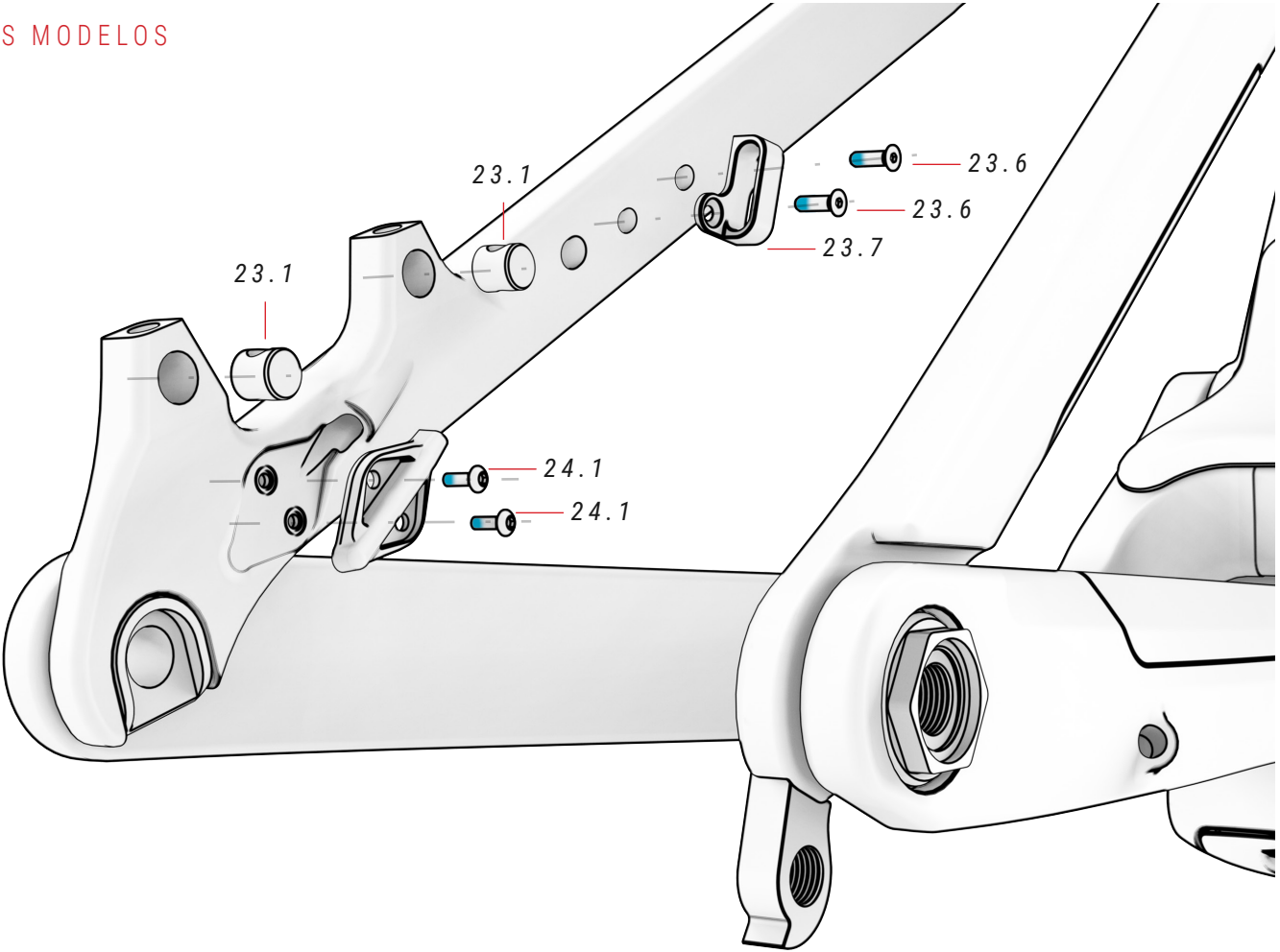
24 TORNILLO SENSOR VELOCIDAD
